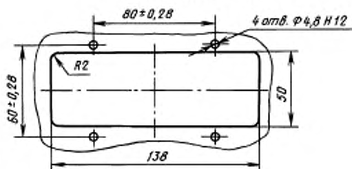
Комплект КЗР
