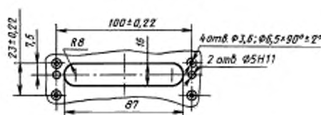
Комплект КЗВ
