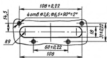
Комплект КЗВ
