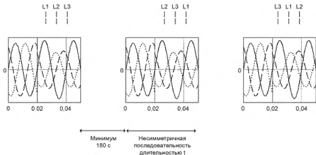
Рисунок 2 — Чередование трех несимметричных испытательных последовательностей (циклический сдвиг напряжений U_a , U_b и U_c )
