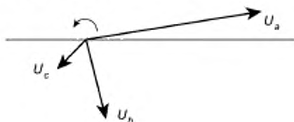
Рисунок A.1 — Несимметричные векторы напряжения
