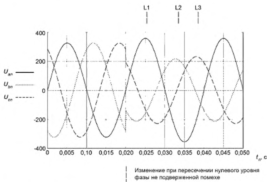
Рисунок 1 — Пример несимметричного трехфазного напряжения питания (испытание 3)
