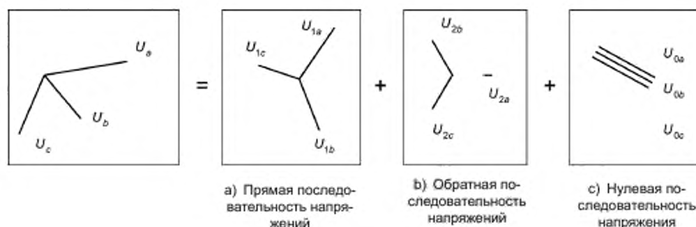
Рисунок A.2 — Составляющие несимметричных векторов на рисунке A.1
