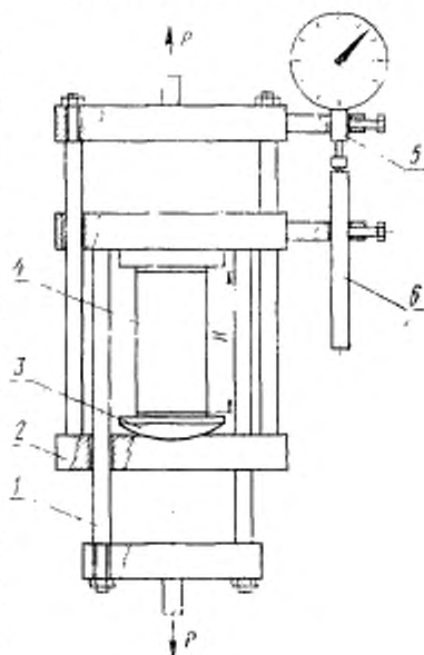
1 — нижняя траверса реперсора; 2 — верхняя траверса реперсора; 3 — шарнирная опора; 4 — образец; 5 — индикатор часового типа; 6 — упорный шток
