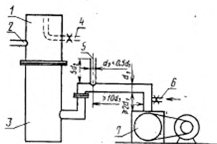
1—измерительная камера; 2, 5—измерительные преобразователи давления; 3—диффузионный насос; 4—клапан V_1 ; 6—клапан V_2 ; 7—механический насос
