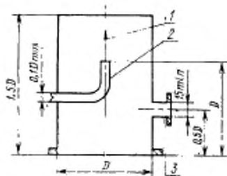
1—направление потока газа; 2—напускная трубка; 3—место подсоединения вакуумметра
