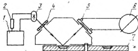
1—стабилизатор напряжения В 2-2; 2—дроссель; 3—бактерицидная лампа ДБ-15; 4—стеклянная пластинка, не пропускающая излучение с длиной волны 253,7 нм; 5—фотоэлемент селеновый с корректирующим фильтром ФЭС-10; 6—гальванометр типа М 195/2; 7—поворотный диск с кюветами для люминофора
