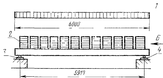
Схема испытания плит
