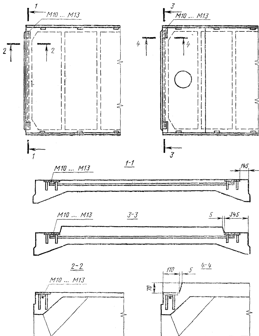
Плита типов ПГ, ПЛ, ПФ
