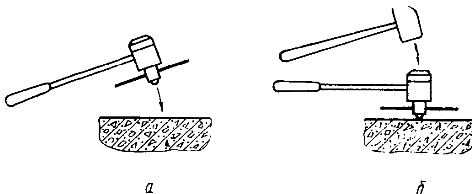
a — нанесение удара эталонным молотком; б — нанесение удара обычным молотком по головке эталонного молотка
