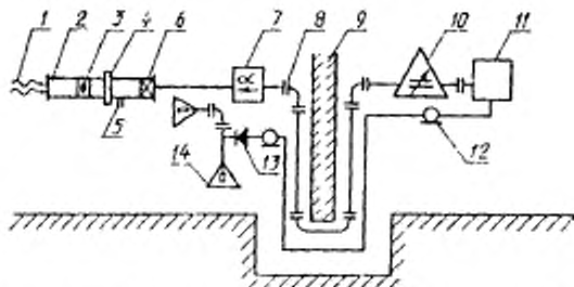
Схема измерений в диапазоне СВЧ
