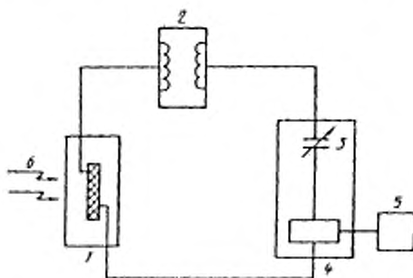
Схема измерений в низкочастотном диапазоне
