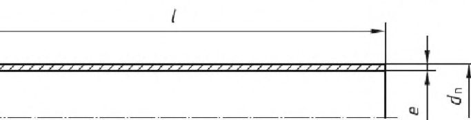
б) Труба без раструба с фаской и без фаски
