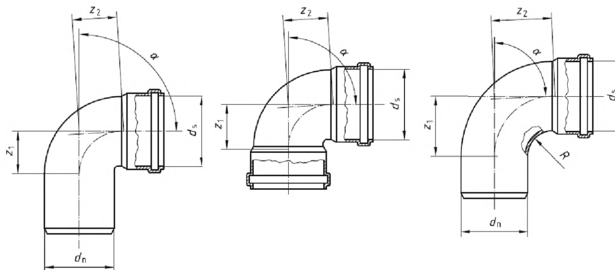
а) Отвод
