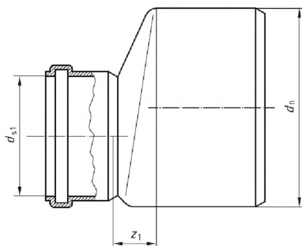
Рисунок 8 – Патрубок переходной
