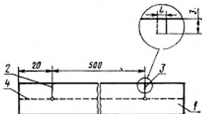
1—образец; 2—первый надрез; 3—второй надрез; 4—шов
