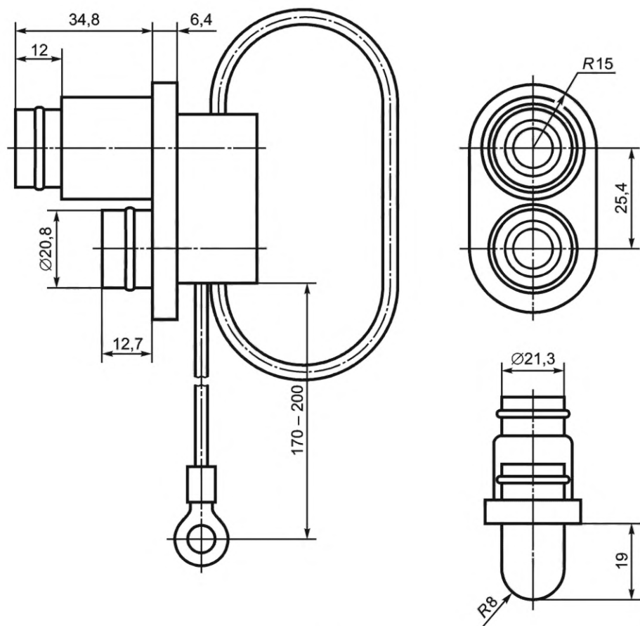
Рисунок 4 — Заглушка
