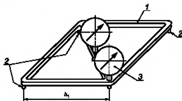
Схема прибора для измерения отклонений от плоскостности
