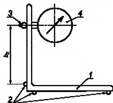
Схема прибора для измерения отклонений от перпендикулярности
