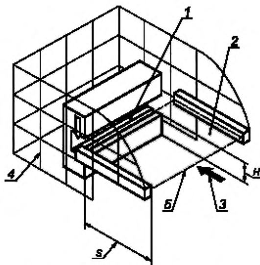
Рисунок 4 — Параллельное приближение к зоне обнаружения
