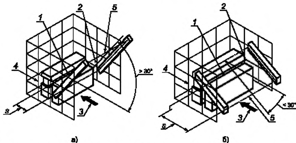
Рисунок 4 — Параллельное приближение к зоне обнаружения
