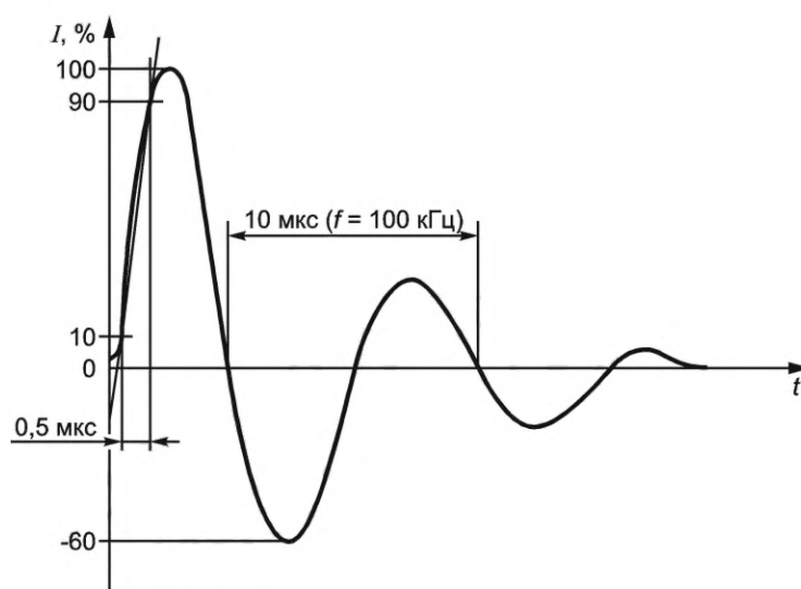
Рисунок 16 — Волна тока импульсного генератора 0,5 мкс/100 кГц
