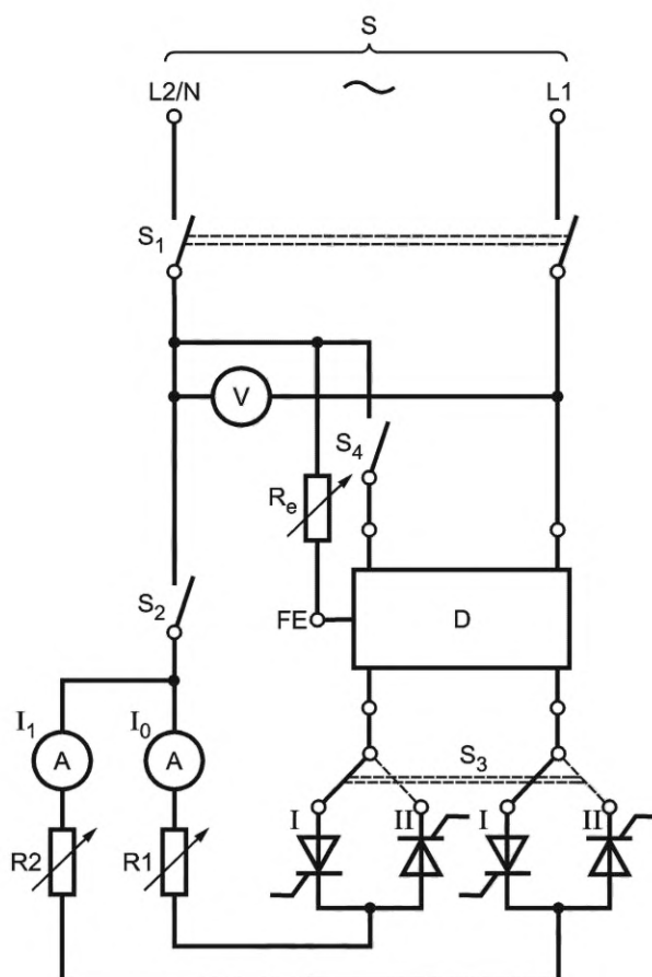
S — подача питания; V — вольтметр; A — амперметр (измеряющий среднеквадратичные значения); D — испытуемое УЗО-Р; R_e — переменный резистор; R_1 — переменный резистор; R_2 — переменный резистор; S_1 — двухполюсный выключатель; S_2 — однополюсный выключатель; S_3 — однополюсный двухпозиционный переключатель; S_4 — однополюсный выключатель; FE — рабочее заземление
