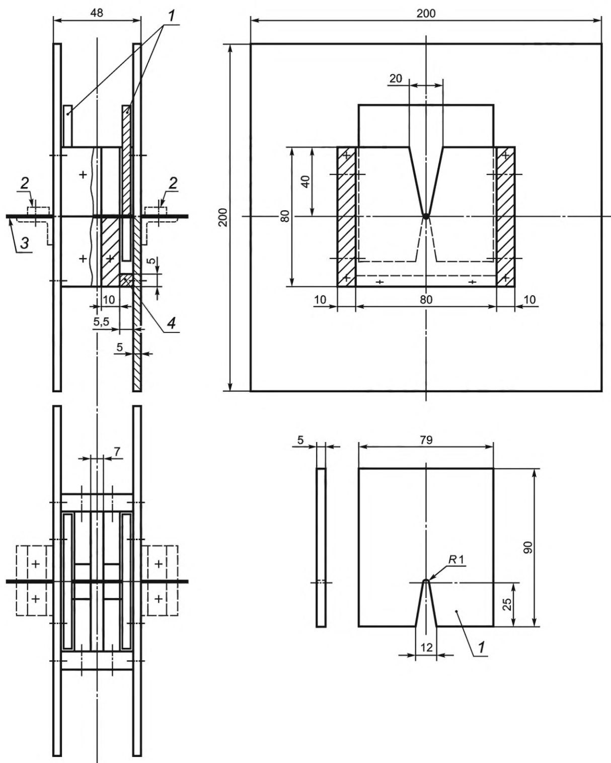
Рисунок 19 — Испытательное устройство для проверки минимальных значений I^2t и I_p , которые должны выдерживать УЗО-Р (перечисление а) 9.15.2.1)
