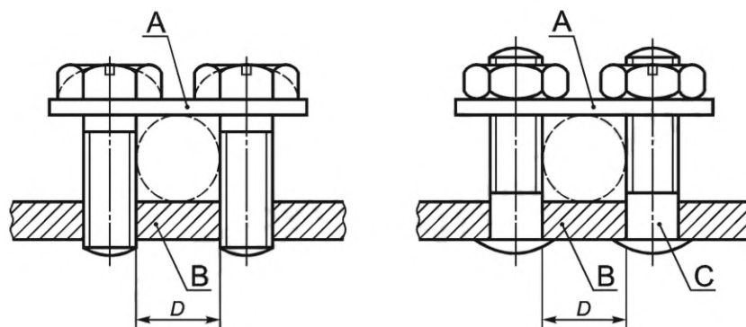
А — седло; В — фиксированная часть; С — винт; D — пространство для проводника
