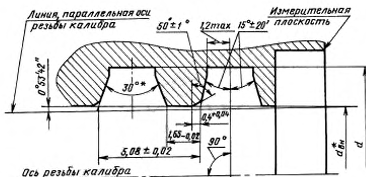
Профиль резьбы калибра-кольца с неполным профилем Р-Н
