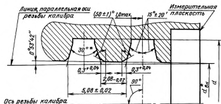
Профиль резьбы калибра-кольца с полным профилем Р-П
