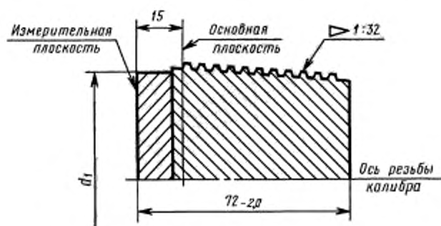
Калибр-пробка Р
