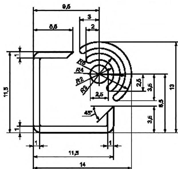
Рисунок В.1 — Структура основы эмблемы радиочастотной идентификации
