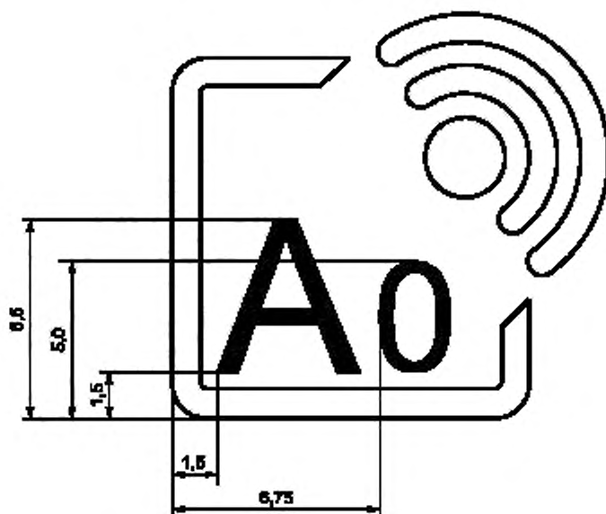
Рисунок В.4 — Эмблема радиочастотной идентификации с двузначным кодом
