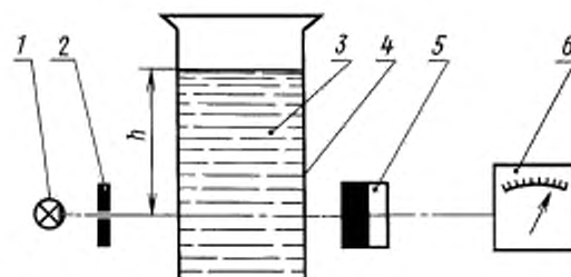
1 — источник света; 2 — диафрагма; 3 — суспензия порошка, 4 — стеклянная кювета; 5 — фотоэлемент; 6 — блок регистрации и записи фотоэлектродвижущей силы (фототока); h — высота оседания частиц порошка
