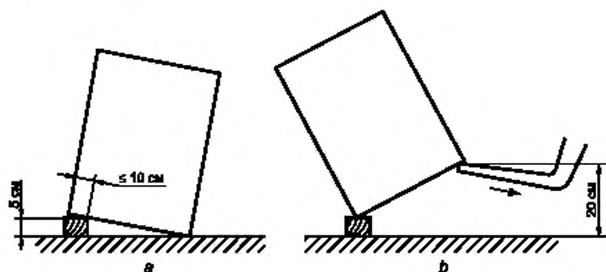
Рисунок 2 — Испытание на сбрасывание плашмя на основание
