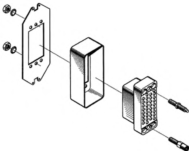
Рисунок 8 – Иллюстрация монтажа соединителя АКД
