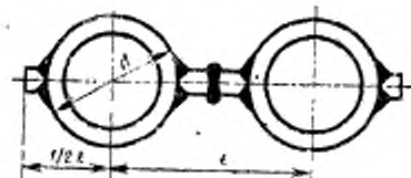
Стенка из плавниковых труб с вваренной между ними вставкой
