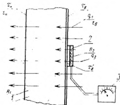
Схема измерения плотности теплового потока
