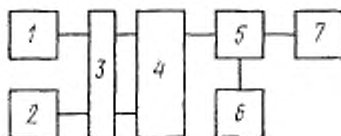
1, 2—источники постоянного оптического излучения; 3—измерительный ослабитель; 4—оптический смеситель; 5—камера с последующим ФЭУ, делителем напряжения питания и резистором анодной нагрузки; 6—источник питания ФЭУ; 7—вольтметр постоянного тока.
