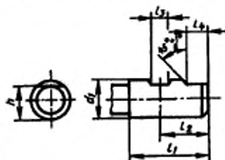
Исполнение 3 для d_1 = 25-63 мм
