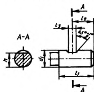
Исполнение 2 для d_1 = 6-20 мм
