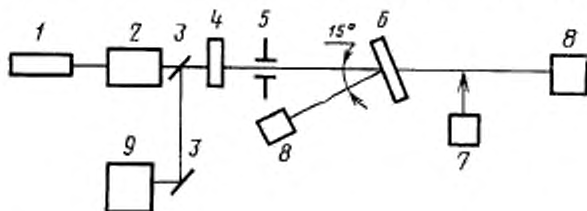
1—юстировочный лазер для измерений на длинах волн 0,69 и 1,06 мкм; 2—лазер для измерений на длинах волн 0,69; 1,06; 10,6 мкм; 3—зеркало; 4—механический затвор для измерений на длине волны 10,6 мкм; 5—диафрагма; 6—делительная пластина; 7—исследуемый преобразователь с системами регистрации и термостатирования; 8—хотрольное средство измерений энергии одиночных импульсов; 9—юстировочный лазер для измерений на длине волны 10,6 мкм
