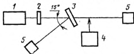
1—блок лазера для измерений на длинах волны 0,6; 0,63 и 10,6 мкм, совмещенного с юстировочным лазером; 2—диафрагма; 3—делительная пластина; 4—исследуемый преобразователь с системами регистрации и термостатирования; 5—контрольное средство измерений средней мощности
