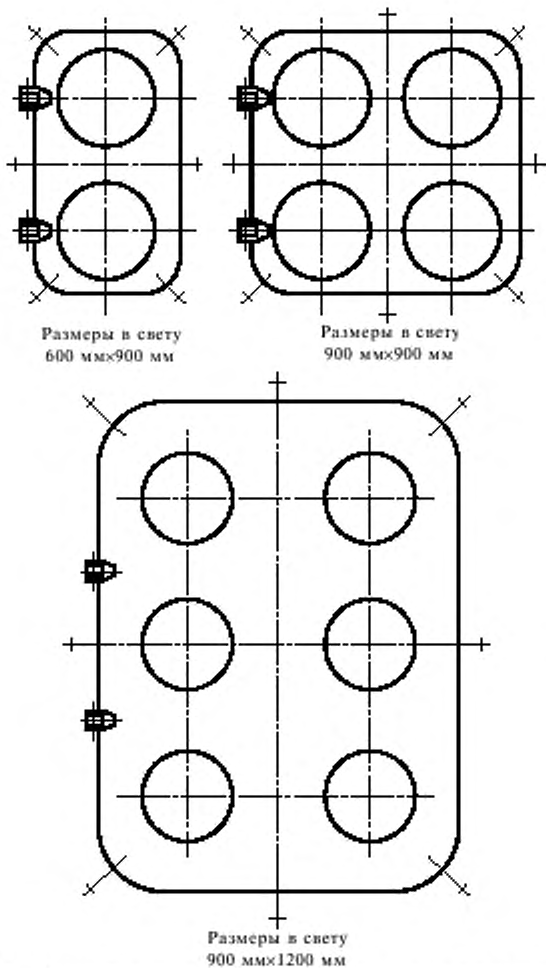
Рисунок 2 — Схемы расположения иллюминаторов, задраск и петель на крышках типа А
