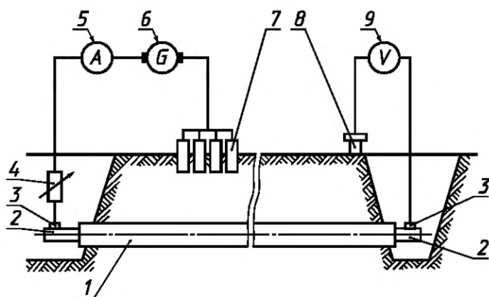
1 — трубопровод; 2 — незаизолированный конец трубопровода; 3 — контакты; 4 — резистор; 5 — амперметр; 6 — источник постоянного тока; 7 — временное анодное заземление; 8 — медно-сульфатный электрод сравнения; 9 — вольтметр
