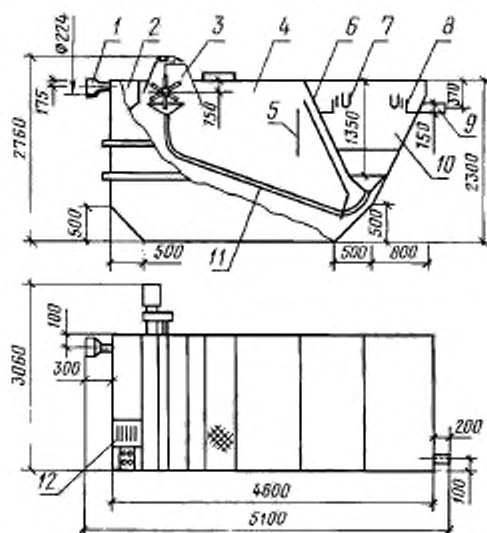
Установка КУ-12
