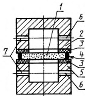
1 — образец; 2 — крышка; 3 — резиновая прокладка; 4 — уплотнение боковой поверхности образца смесью, состоящей из 60% парафина и 40% канцфолы, синтетической смолы или другого уплотнителя; 5 — основание; 6 — каналы диаметром от 1,5 до 2,0 мм для отвода и манометр газа или жидкости; 7 — каналы для подвода и отвода жидкости или газа
