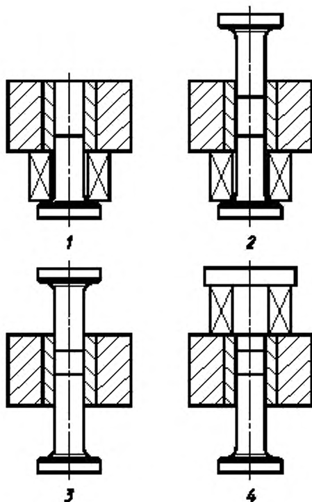
1 — загрузка; 2 — предварительное прессование; 3 — прессование; 4 — выпрессовывание
