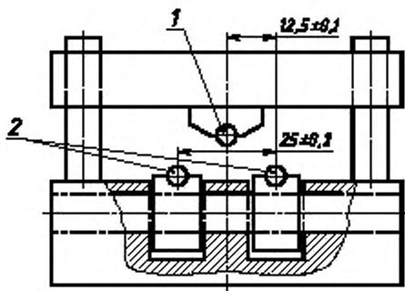
1 — нагрузочный ролик, 2 — опорный ролик
