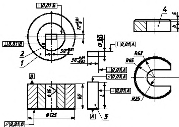
1 — обойма; 2 — матрица; 3 — пуансоны; 4 — опоры
