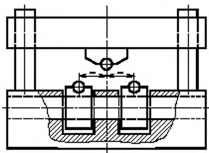
Рисунок А.2 — Схема устройства для испытания
