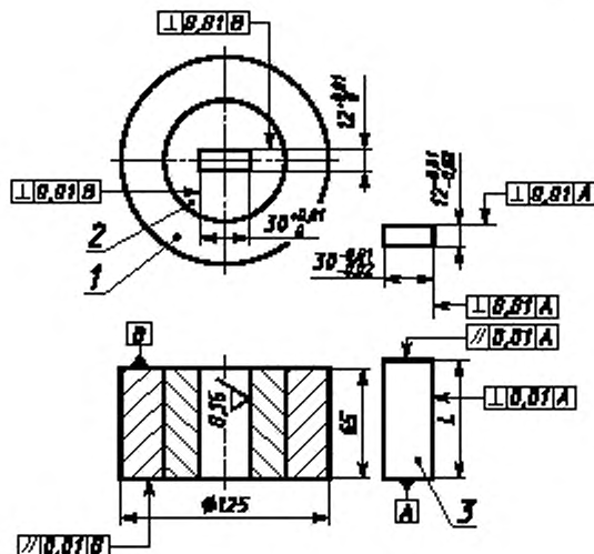
Рисунок А.1 — Пресс-форма для прессования прямоугольных образцов
