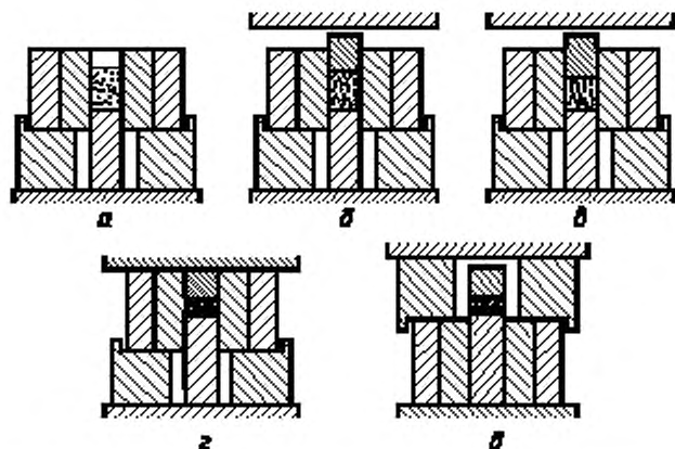
а — загрузка порошка в пресс-форму б — установка верхнего пуансона; в — предварительное прессование г — замена опоры и окончательное прессование д — вытягивание
