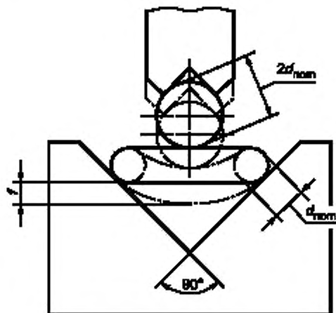
Рисунок 1 — Прогиб f
