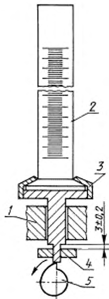
1 — направляющий подшипник, 2 — градуированный измерительный цилиндр, 3 — держатель с направляющим штырем 4 — опора (стальная); 5 — кулачок
