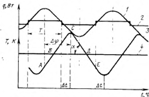
1, 2—кривые наращения мощности, вводимой в образец; 3—кривая колебания температуры на поверхности образца, 4—средняя установившаяся температура образца.
