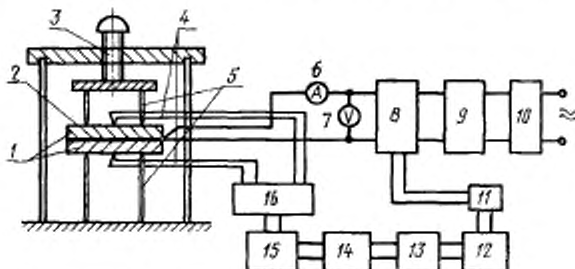
1—исследуемый образец; 2—нагреватель; 3—прижимной винт; 4—термометр; 5—держатель; 6—миллиамперметр; 7—вольтметр; 8—электромагнитное реле; 9—генератор; 10—выпрямитель; 11—реле; 12—самовсеч электронный; 13—усилитель; 14—магазин сопротивлений; 15—потенциометр; 16—переключатель
