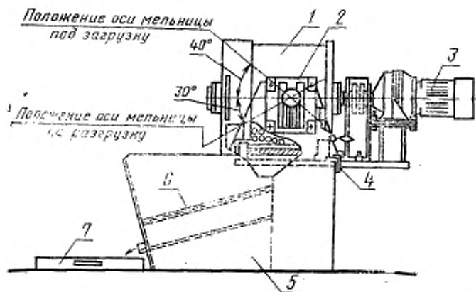
1—барабан; 2—ручной редуктор для поворота мельницы; 3—электродвигатель; 4—фиксатор положения мельницы; 5—приемный сосуд; 6—дно из сетки; 7—протазна
