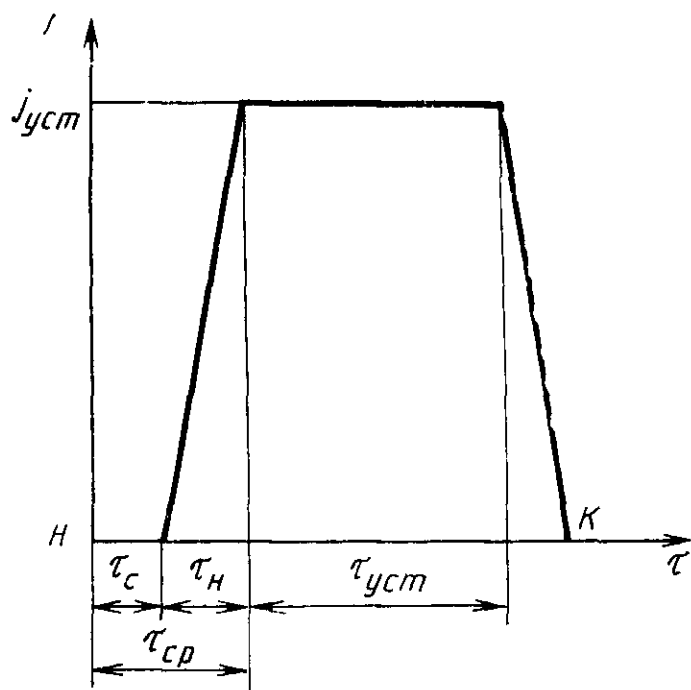
Схема тормозной диаграммы
