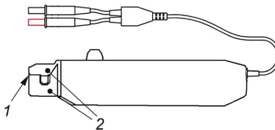
Тип D — датчик тока для НЕОПАСНЫХ для ЖИЗНИ применений (показан со скользящим ЗАЖИМОМ)
