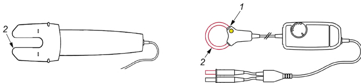
Тип А — датчик тока с ЗАЖИМОМ в форме вилки
