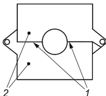
Тип С — датчик тока с разделенным сердечником
