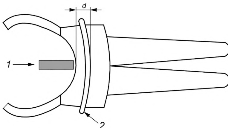
1 — ОПАСНЫЙ проводник, находящийся под НАПРЯЖЕНИЕМ; 2 — ЗАЩИТНЫЙ БАРЬЕР; d — расстояние между ЗАЩИТНЫМ БАРЬЕРОМ и ОПАСНЫМ проводником, находящимся под НАПРЯЖЕНИЕМ
