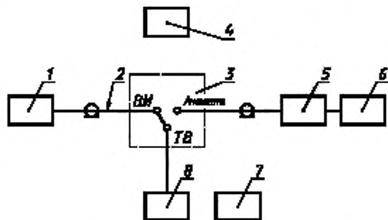
1 — ВИ; 2 — соединительный кабель, входящий в комплект ВИ; 3 — антенный переключатель, входящий в комплект ВИ; 4 — генератор замещающих сигналов; 5 — согласующий attenuator; 6 — измеритель радиопомех; 7 — контрольный ТВ (монитор); 8 — эквивалент нагрузки сопротивлением 75 Ом
