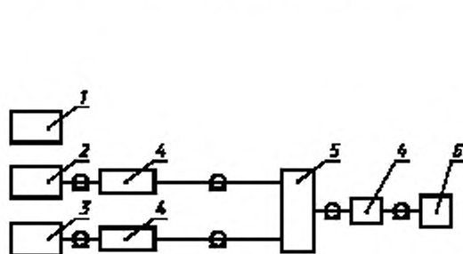
1 — генератор замещающих сигналов; 2 — испытуемое устройство; 3 — генератор испытательных сигналов; 4 — согласующий attenuator; 5 — разветвитель; 6 — измеритель радиопомех
