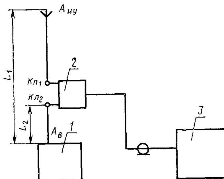
1 — испытуемый приемник; 2 — измерительное устройство (п. 3.1 настоящего приложения); 3 — измеритель радиопомех (п. 2.2.3 настоящего стандарта)
