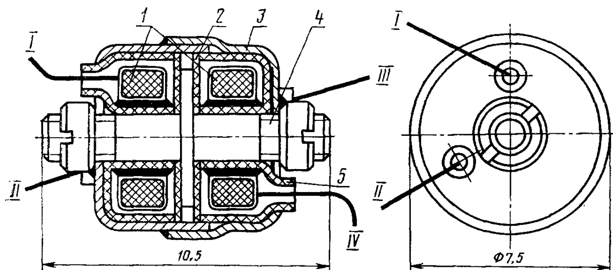
1 — тороидальный ферритовый сердечник; 2 — крышка из полиэтиленовой пленки; 3 — внешний экран; 4 — шпилька-экран; 5 — корпус из сополимера; I, II — выводы первичной обмотки трансформатора; III, IV — выводы вторичной обмотки трансформатора
