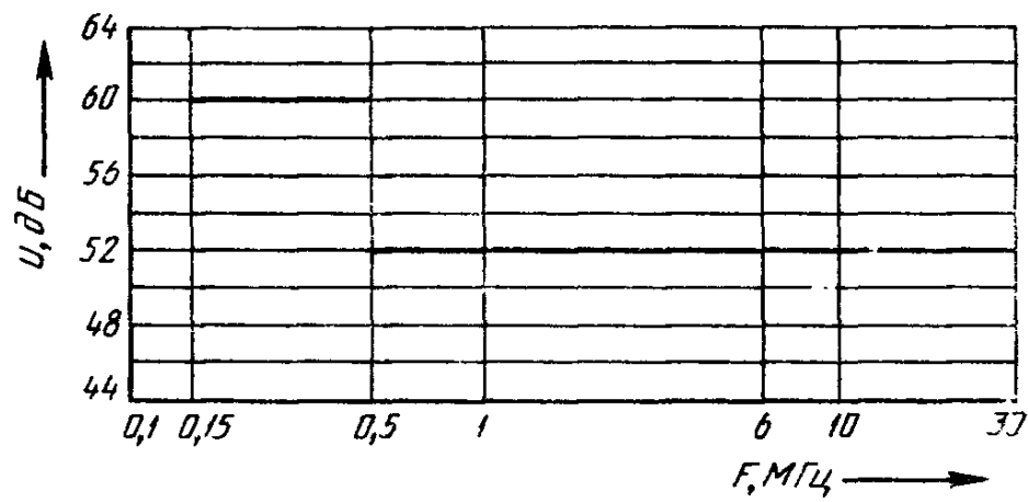
U — напряжение радиопомех; F — частота Черт. 1а
