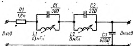
Электрическая схема фильтра нижних частот
