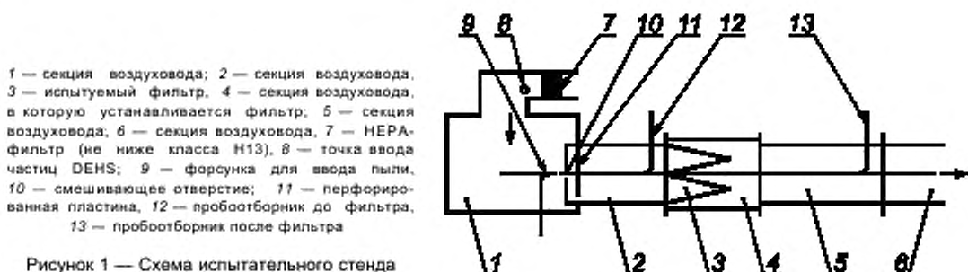
Рисунок 1 — Схема испытательного стенда
