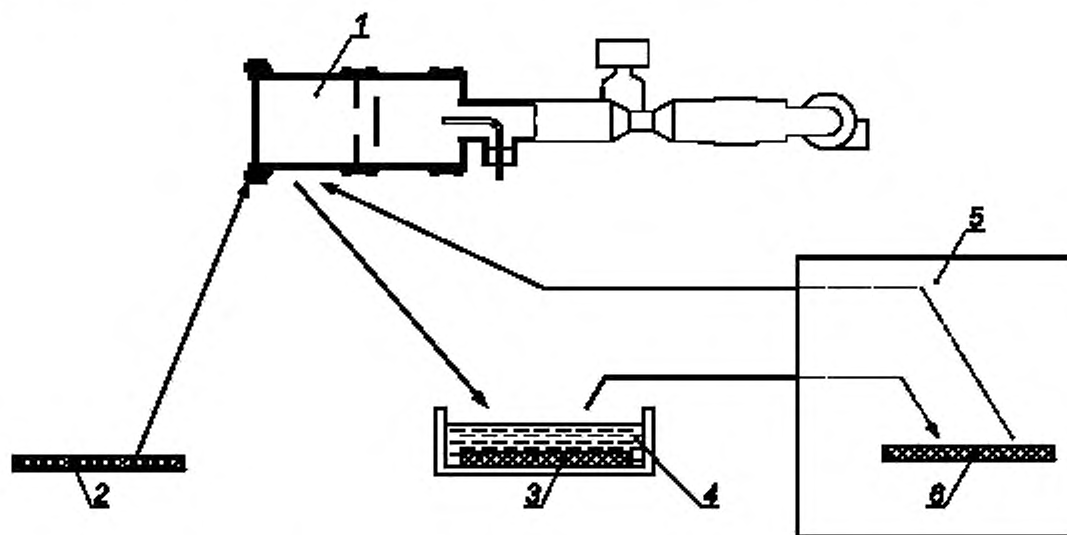
1 — устройства для измерения эффективности; 2 — образец фильтрующего материала; 3 — обработка изопропанолом; 4 — ювета (емкость) с изопропанолом; 5 — вытяжной шкаф; 6 — сушка образца материала
