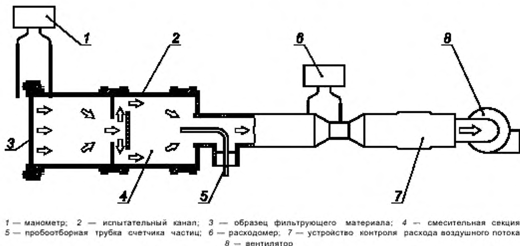
Рисунок А.1 — Оборудование для испытаний фильтрующего материала
