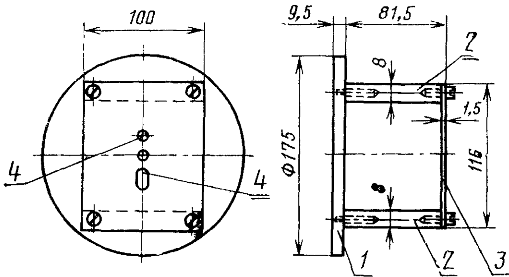
1 — деревянная крепежная плита, 2 — алюминиевые плиты, 3 — сменная стальная плита; 4 — отверстия для крепления образца
