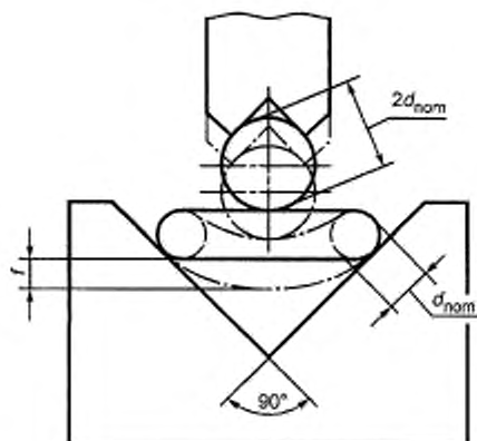
Рисунок 1 — Прогиб f
