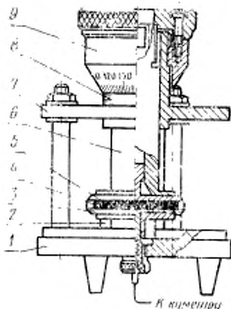
1 — нижнее основание; 2 — фарфоровый фторопластовый изолятор; 3 — нижняя обкладка измерительного конденсатора; 4 — образец; 5 — верхняя подвижная обкладка измерительного конденсатора; 6 — подвижной шток микрометрического винта; 7 — верхняя плата; 8, 9 — микрометрический винт
