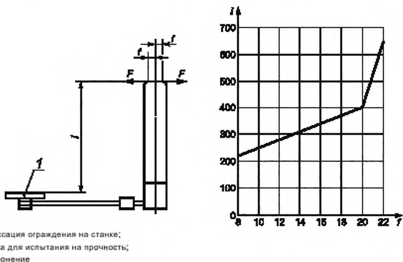
Рисунок А.1 — Наибольшая величина упругой деформации ограждения, при испытании ограждения «мостового типа»
