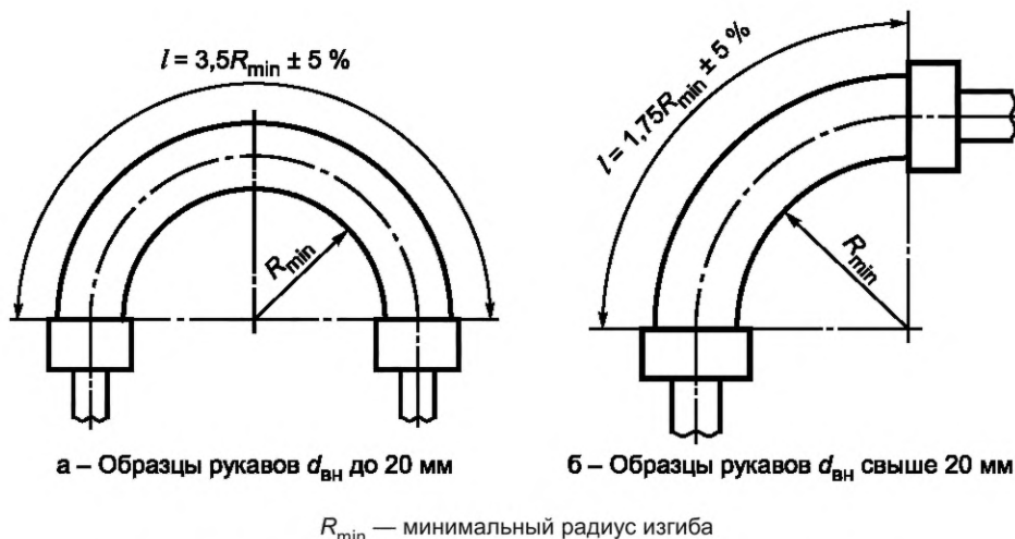
Рисунок 3 — Схема изгиба рукавов при динамических испытаниях
