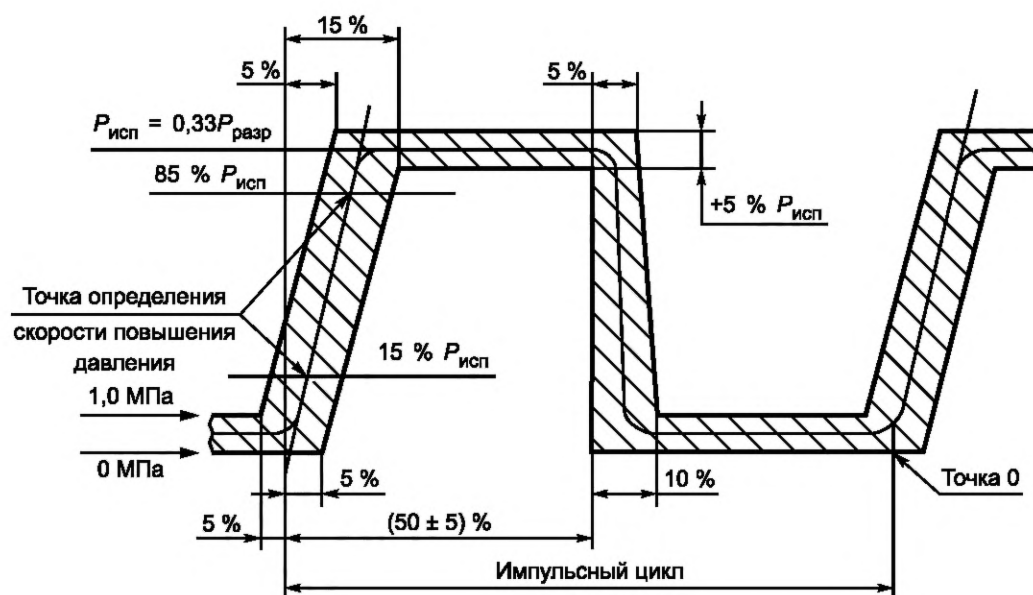
Рисунок 2 — Импульсный цикл динамического испытания рукавов
