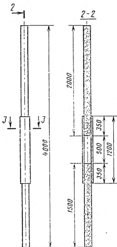
Опора типа 3
