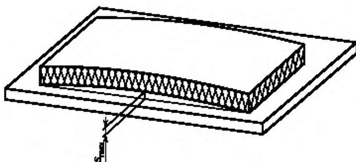
a) Измерение отклонения от плоскостности по длине
