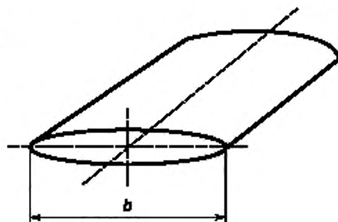
Рисунок 1 — Измерение ширины трубчатых изделий
