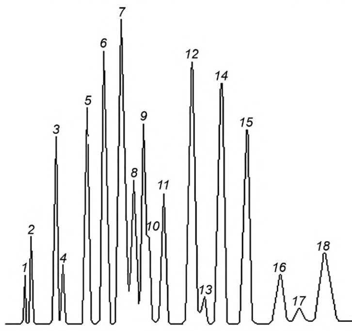
Рисунок Б.11 — Типовая хроматограмма углеводородов C_1 — C_5 на колонке с Al_2O_3/BM
