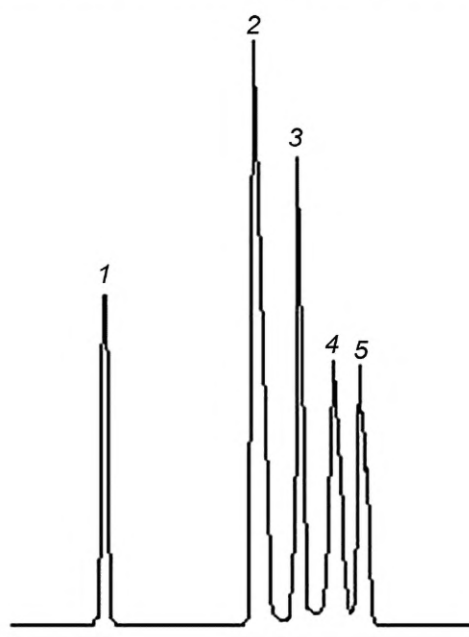
Рисунок Б.1 — Типовая хроматограмма пропановой фракции на колонке с ТЗК/ВМ
