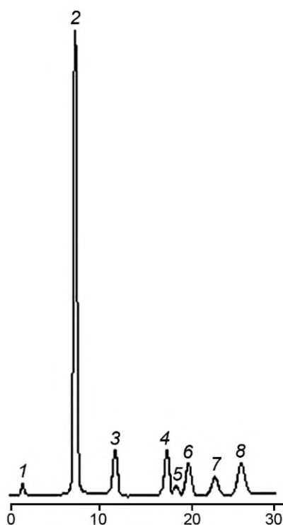
Рисунок Б.8 — Типовая хроматограмма изобутановой фракции на колонке с \text{Al}_2\text{O}_3/\text{BM}
