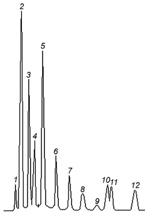
Рисунок Б.9 — Типовая хроматограмма фракции n -Бутана на колонке с \text{Al}_2\text{O}_3/\text{BM}
