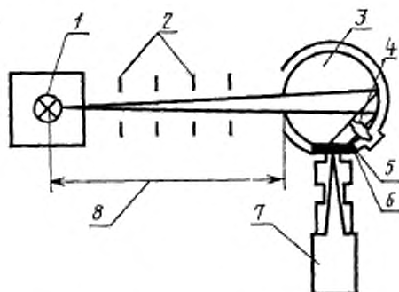
1 — измерительный источник излучения; 2 — диафрагма; 3 — интегрирующая сфера; 4 — затенитель; 5 — образец фотоматериала; 6 — прижимная пластина; 7 — физический приемник; 8 — расстояние от источника света до входного отверстия сферы
