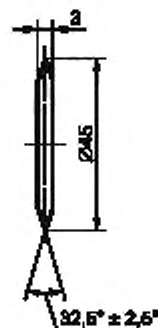
Рисунок 3 — Характеристики круглого лезвия для испытания
