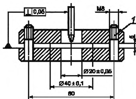
Рисунок 8 — Устройство для крепления образца
