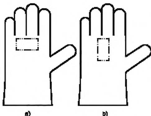
Рисунок 6 — Направление выреза образцов для испытания
